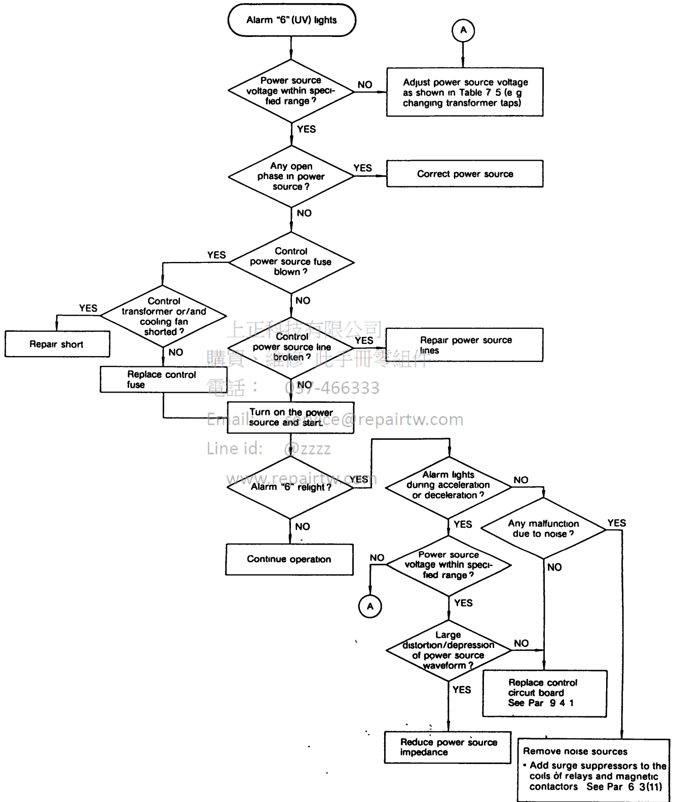
Fig. 9.12 Alarm "6" (UV)
